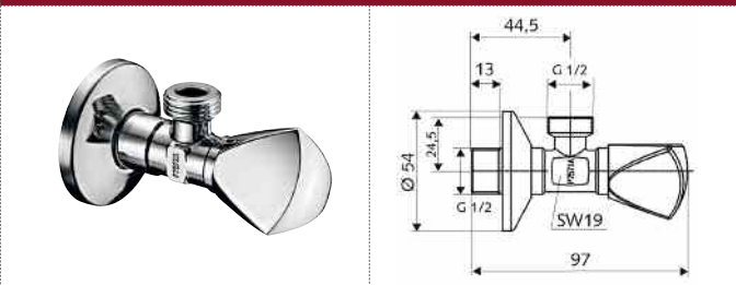
05 276 06 99 SCHELL llave Comfort
