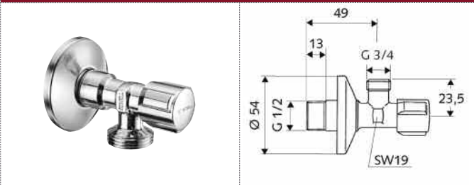
05 406 06 99 SCHELL llave de escuadra segura.
