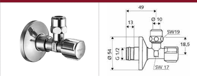
05 152 06 99 SCHELL llave Rondo
