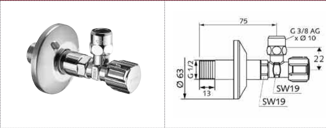
04 925 06 99 SCHELL llave Comfort con vaciador.
