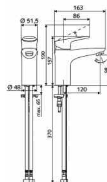
02 182 06 99 SCHELL Modus EH-T maneta plana. 02 183 06 99 SCHELL Modus EH maneta plana.
