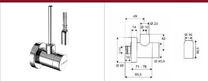
05 172 06 99 SCHELL llave Classic
