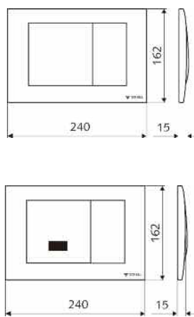
03 126 06 99, 03 126 64 99 SCHELL FIELD y 03 123 06 99 SCHELL FIELD E
