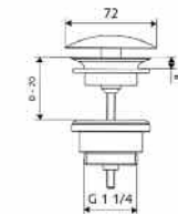
02 002 06 99 SCHELL válvula de desagüe libre.
