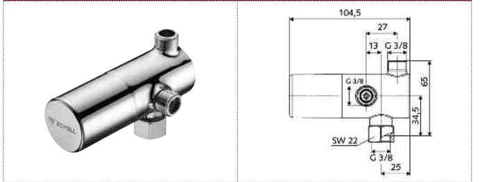
19 114 06 99 SCHELL llave de regulación empotrada.
