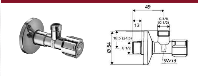
05 430 06 99 SCHELL llave de escuadra con filtro.
