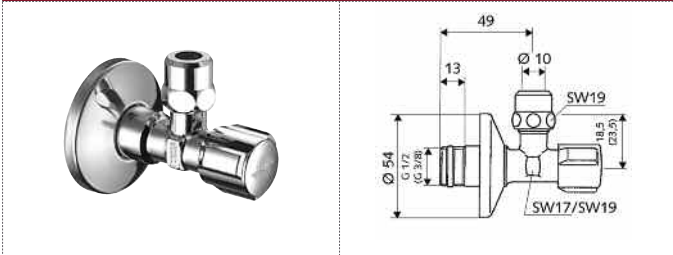
05 217 06 99 SCHELL llave Comfort
