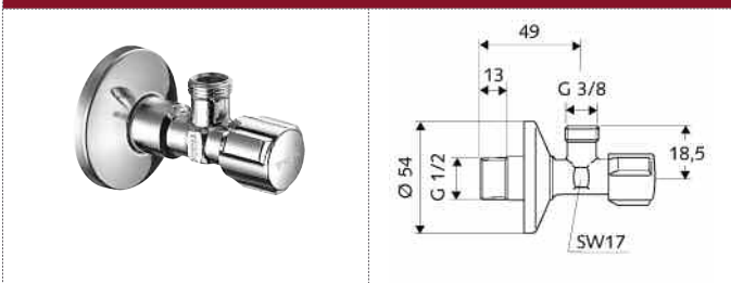
04 907 06 99 SCHELL llave Comfort con tuerca de compresión
