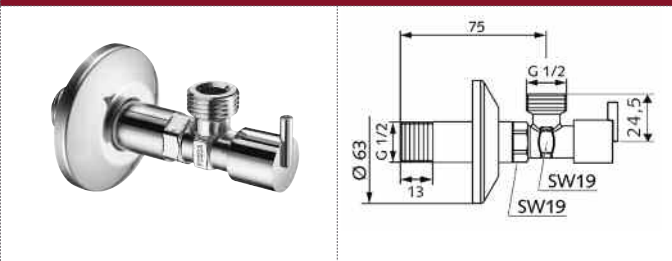
05 418 06 99 SCHELL llave Comfort.
