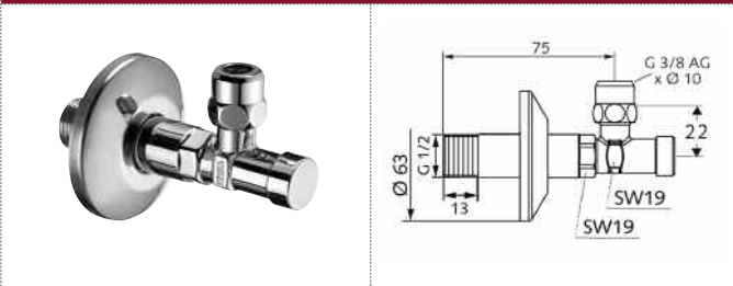
05 405 06 99 SCHELL llave de escuadra segura.
