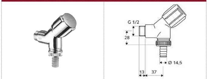
03 386 06 99 SCHELL llave Comfort inclinada para conexión de manguera.
