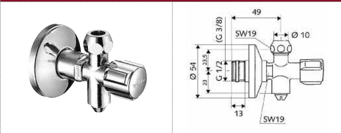
03 300 06 99 SCHELL llave COMFORT.
