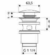
02 002 06 99 SCHELL válvula de desagüe libre.
